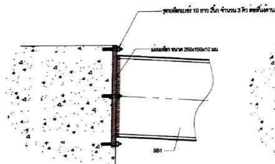
แบบขยาย ① 1:5
