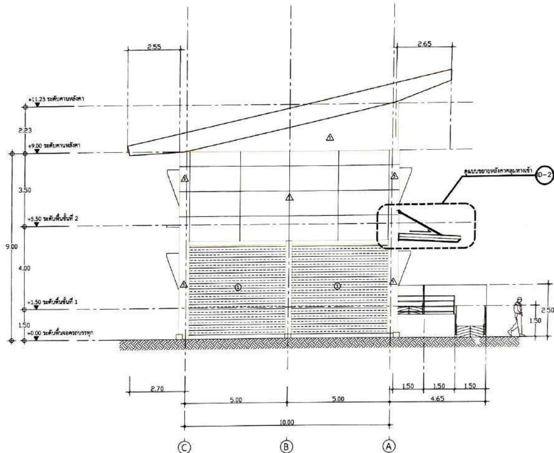
รูปด้าน 2 SCALE 1:125
