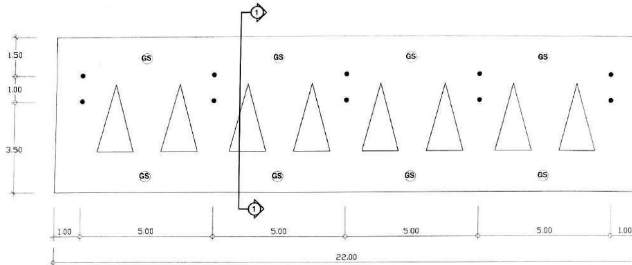
แปลนพื้นโรงจอดรถ
