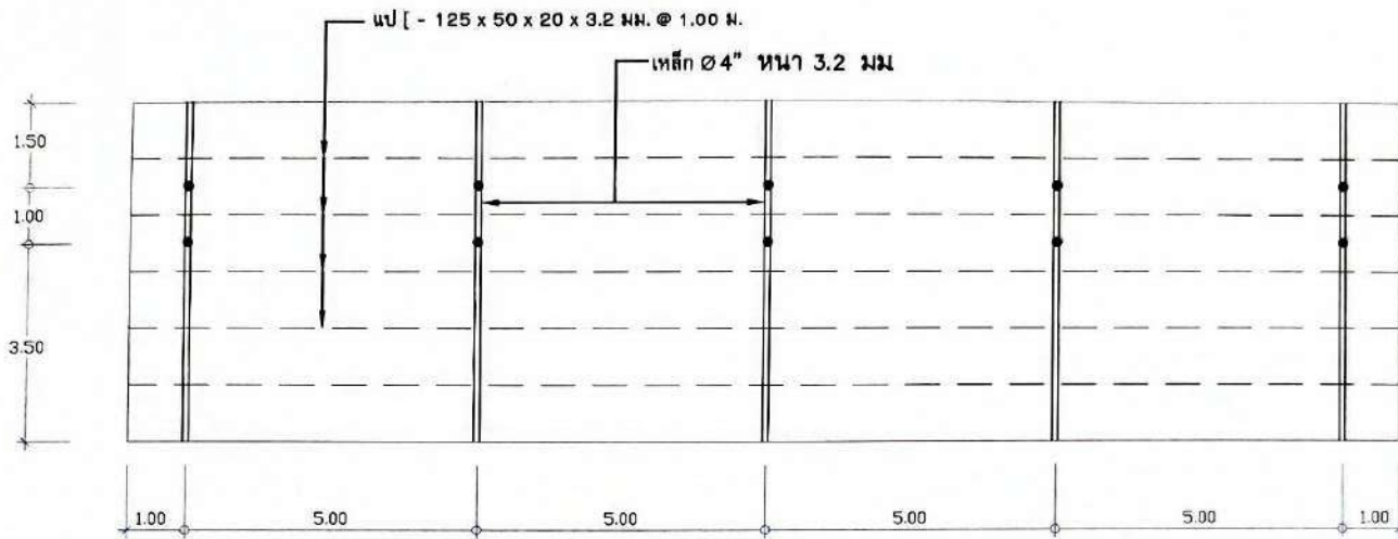
แปลนโครงสร้าง มาตราส่วน 1: 100
