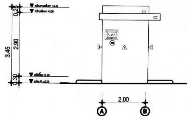
รูปด้าน 4 หน้าอาคาร
