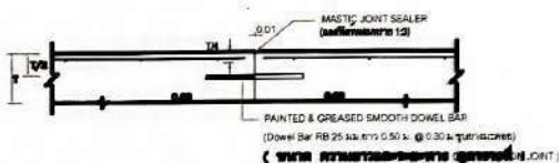
ตารางที่ 2 TIE BARS-DOWEL BARS
