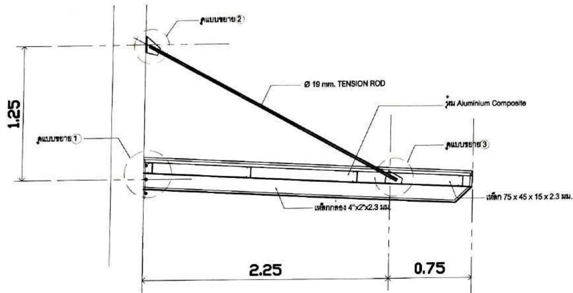
แบบขยายการติดตั้งกันสาด
