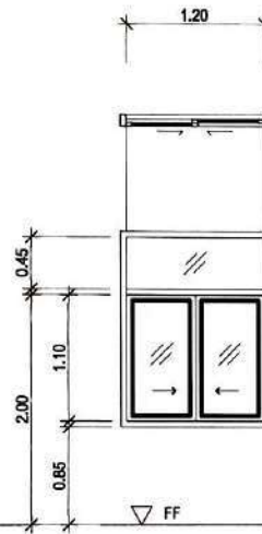
ขยายหน้าต่าง ② มาตราส่วน 1 : 50
