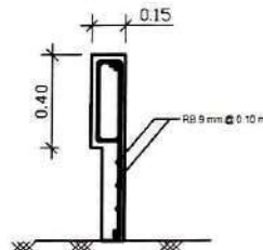
ขยายคาน คอล. SCALE 1:20
