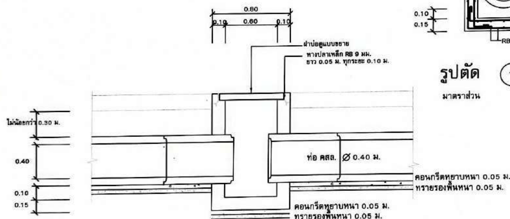
รูปตัด 2 - 2 มาตรฐาน NTS
