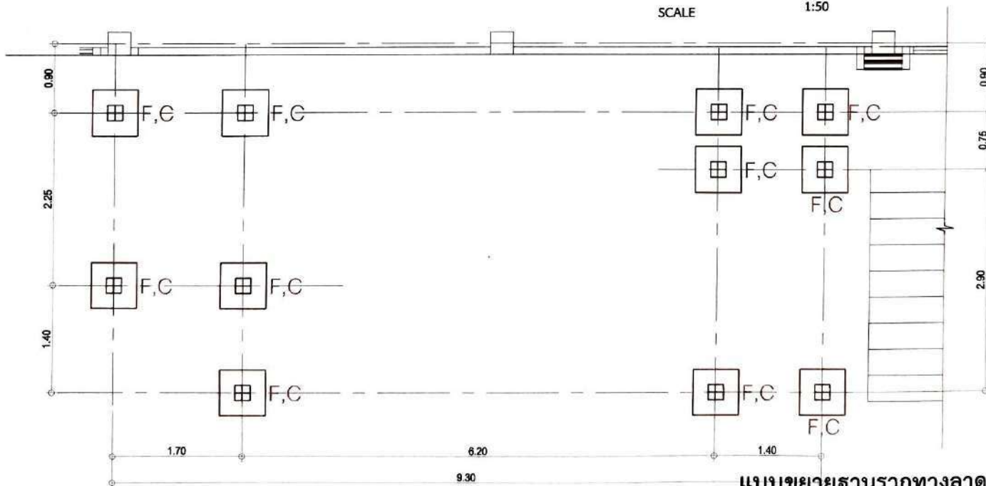
แบบขยายฐานรากทางลาด
