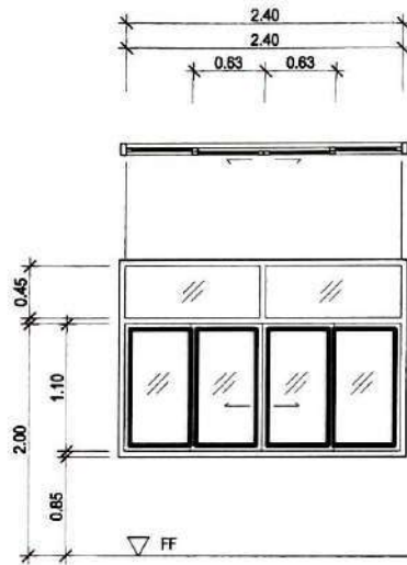
ขยายหน้าต่าง ① มาตราส่วน 1 : 50
