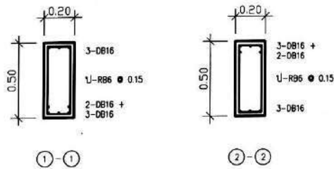
B5 Scale 1 : 25
