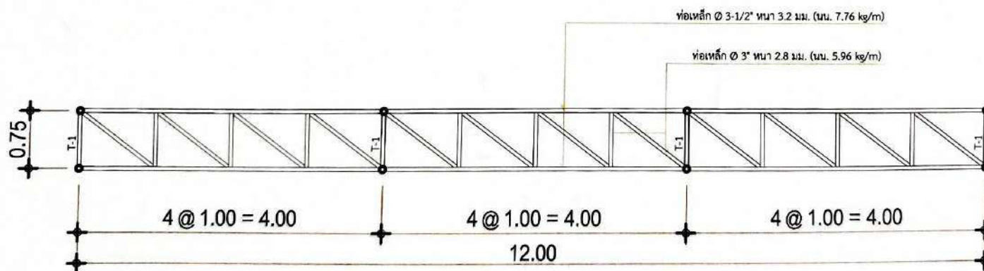
ขยายโครงถัก T2 SCALE 1:50
