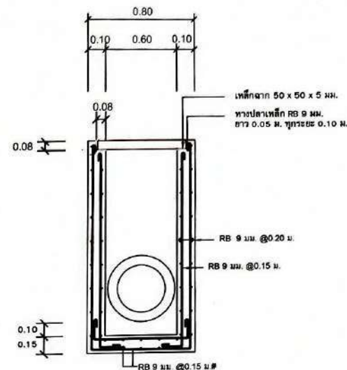
รูปตัด 1 - 1 มาตรฐาน NTS
