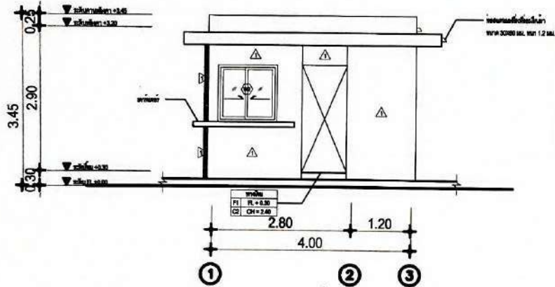
รูปด้าน 1 หน้าอาคาร
