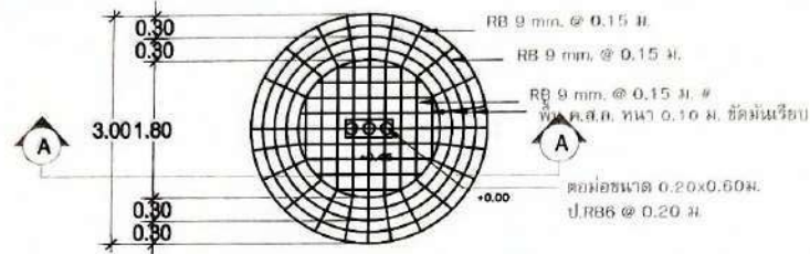
แบบขยายโครงสร้าง Scale 1:75
