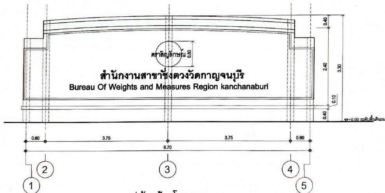
รูปด้านป้ายโครงการ
