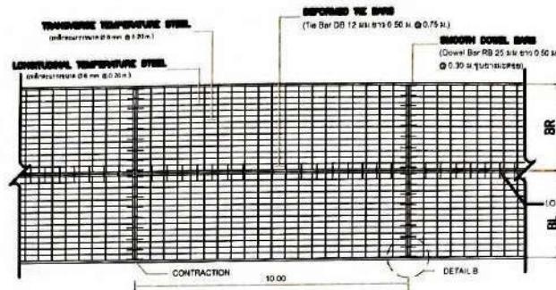
แบบแปลนแสดงการเสริมเหล็กพื้นถนนและลาน คสล. มาตราส่วน 1:20
