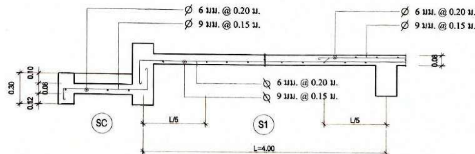
แบบขยายพื้น S1 SCALE 1:25
