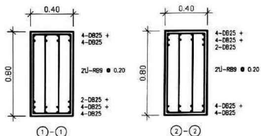
B1 Scale 1 : 25
