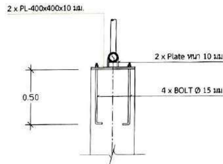
ขยายทิวเสา
