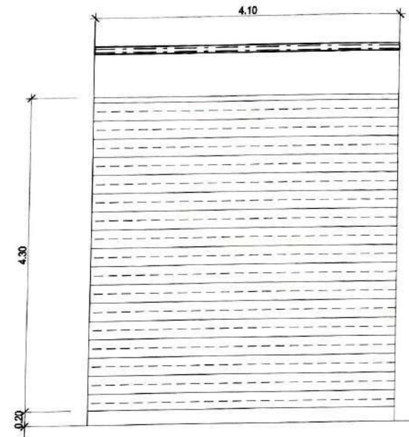
ขยายประตู ② มาตราส่วน 1:50 ประตูบานเหล็กบาน ขนาด 4.10 x 4.30 ม. (มอดอร์ไฟฟ้า)
