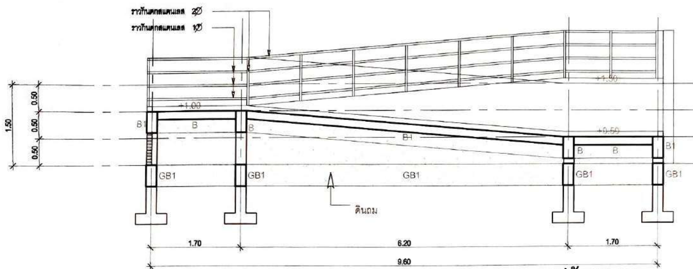
รูปตัดทางลาด SCALE 1:50
