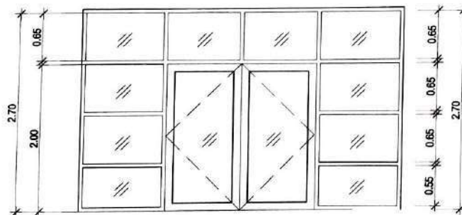
ขยายประตู ② มาตราส่วน 1:50
