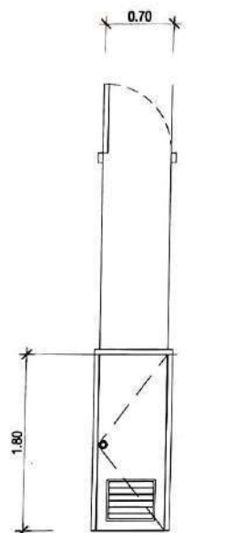
ขยายประตู ④ มาตราส่วน 1 : 50
