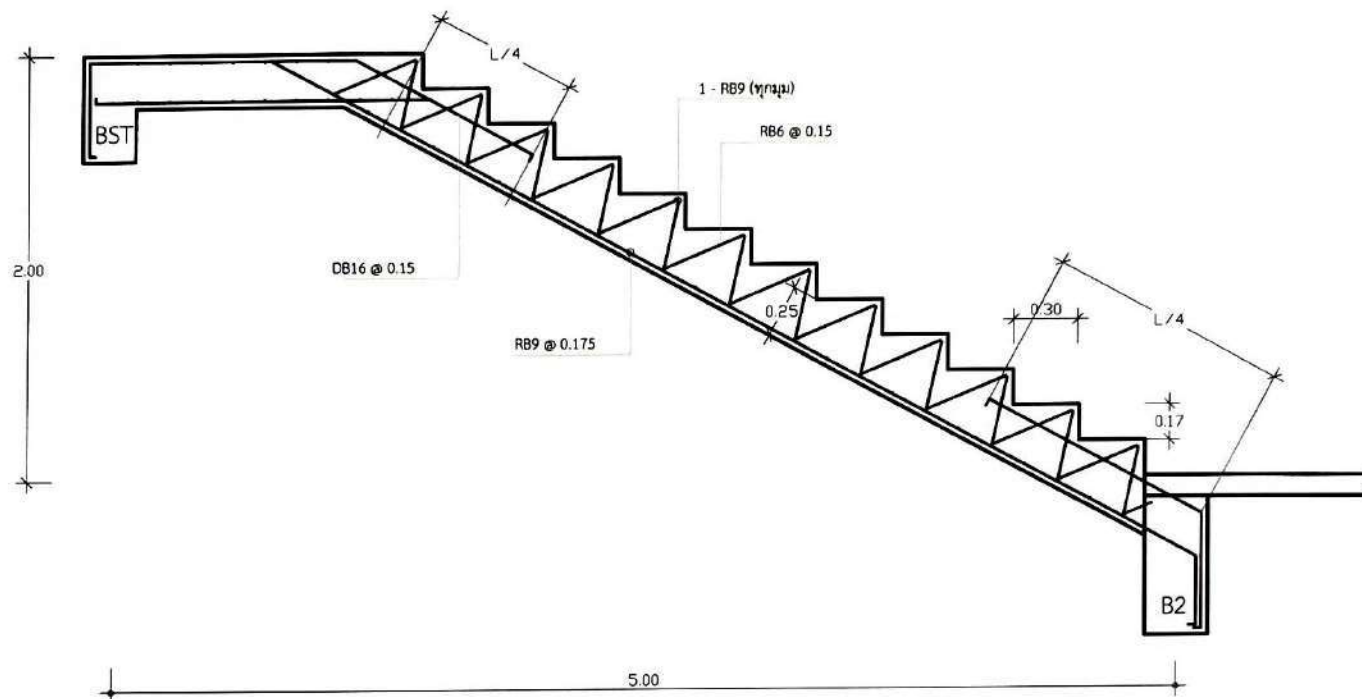
ขยายบันได ST-1
