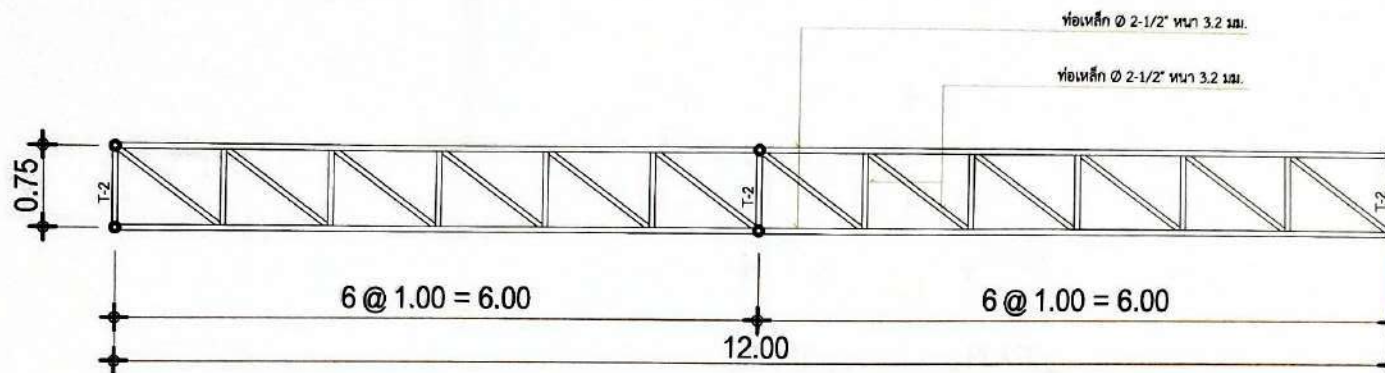
ขยายโครงถัก T1 SCALE 1:50
