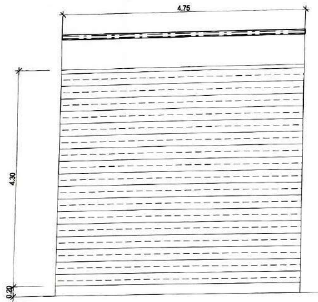
ขยายประตู ① มาตราส่วน 1:50 ประตูบานเหล็กบาน ขนาด 4.75 x 4.30 ม. (มอดอร์ไฟฟ้า)
