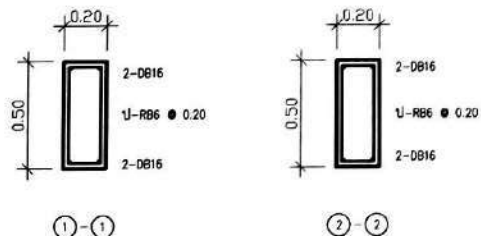
B7 Scale 1 : 25
