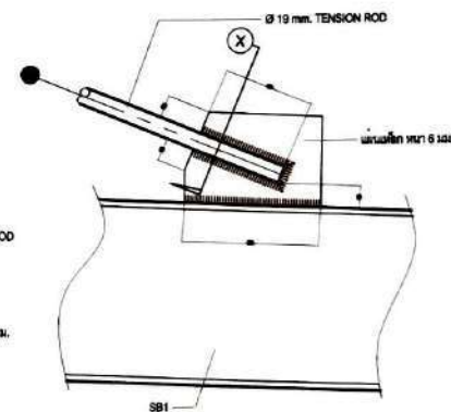
แบบขยาย ③ 1:5
