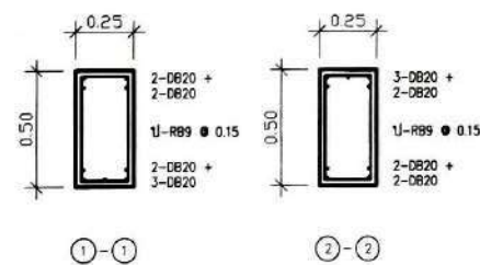
B3, ? BST Scale 1 : 25
