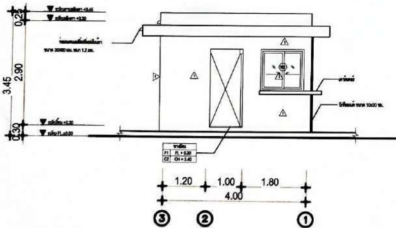
รูปด้าน 3 หน้าอาคาร
