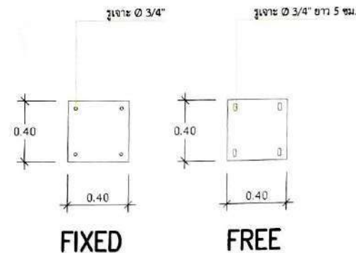
ขยายแผ่นเหล็กรองหัวเสา
