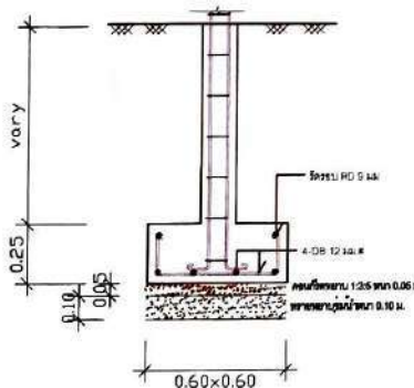
ขยายคานเสา F SCALE 1:20
