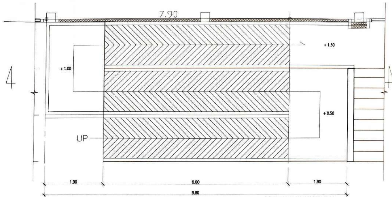
แบบขยายทางลาด
