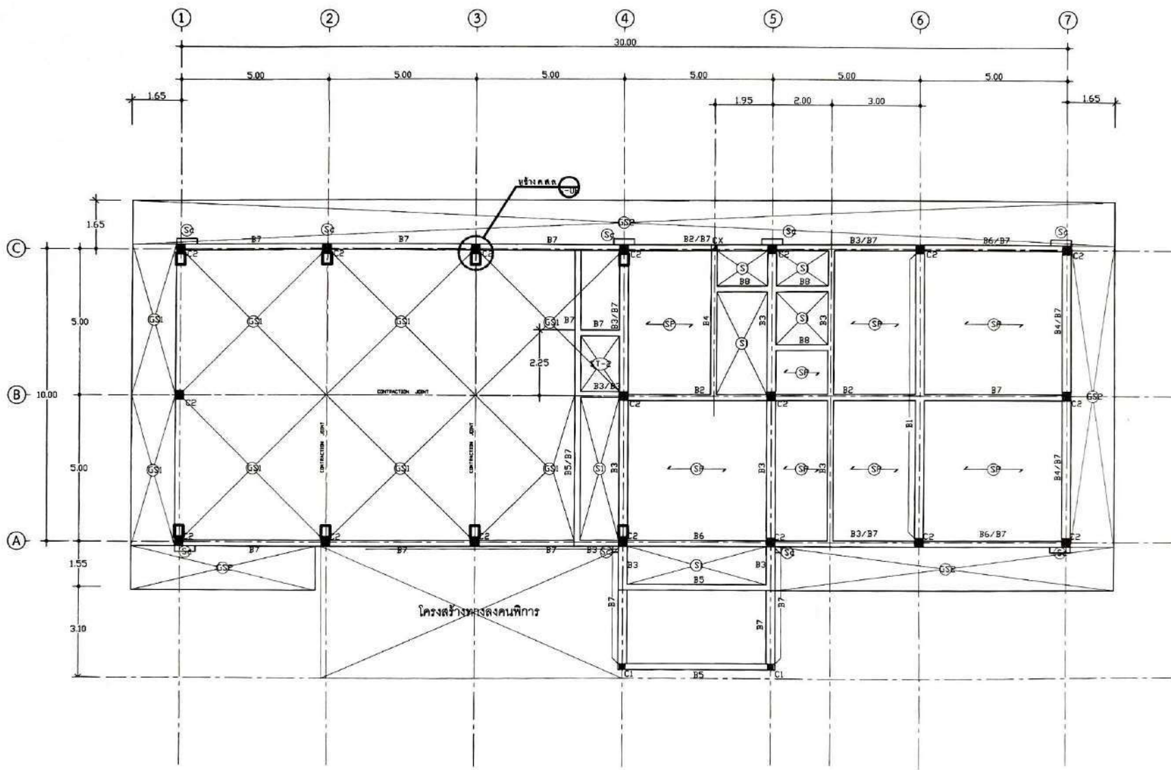
แปลนคานชั้นที่ 1 SCALE 1:125
