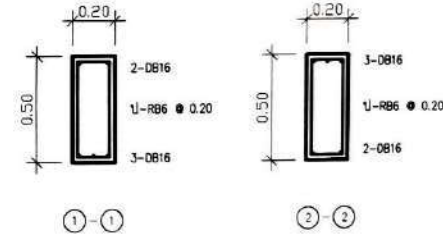
B6 Scale 1 : 25
