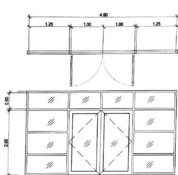
ขยายประตู ③ มาตราส่วน 1 : 50
