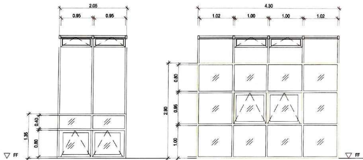
ขยายหน้าตัด ④ มาตราส่วน 1 : 50
