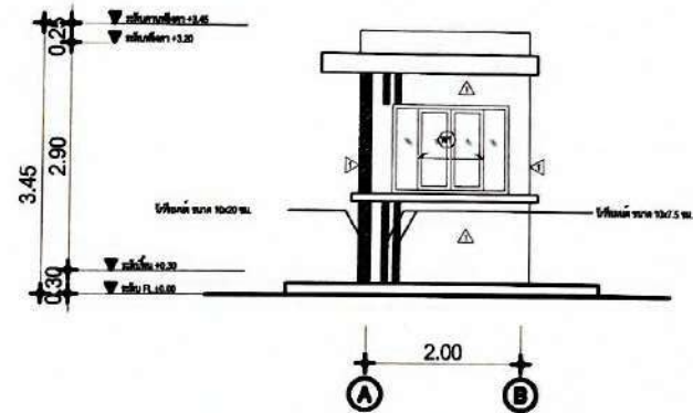
รูปด้าน 2 หน้าอาคาร
