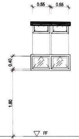
ขยายหน้าต่าง ③ มาตราส่วน 1 : 50
