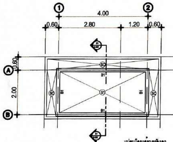
แปลนโครงสร้างหลังคา ขนาดพื้นที่ 1/75
