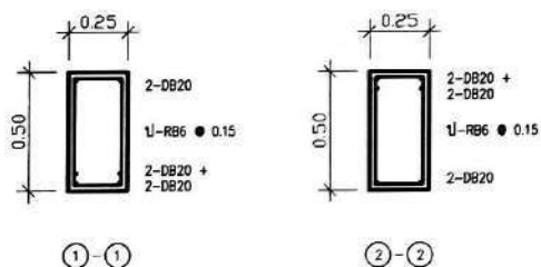
B4 Scale 1 : 25
