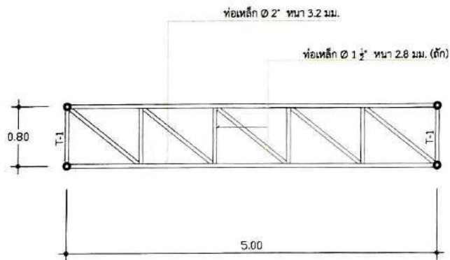
ขยายโครงถัก T-2
