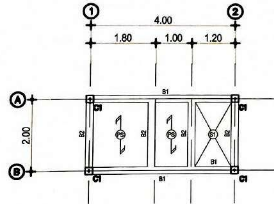
แปลนโครงสร้างพื้น ขนาดพื้นที่ 1/75
