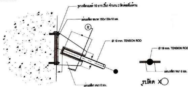
แบบขยาย ② 1:5
