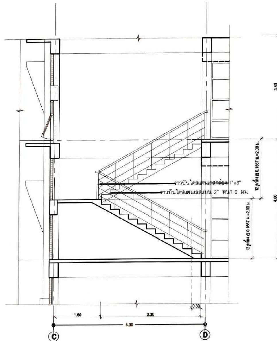
แบบแสดง รูปตัด D-D มาตราส่วน 1:50
