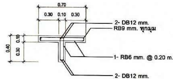
แบบขยายเคาท์เตอร์ SCALE 1:25
