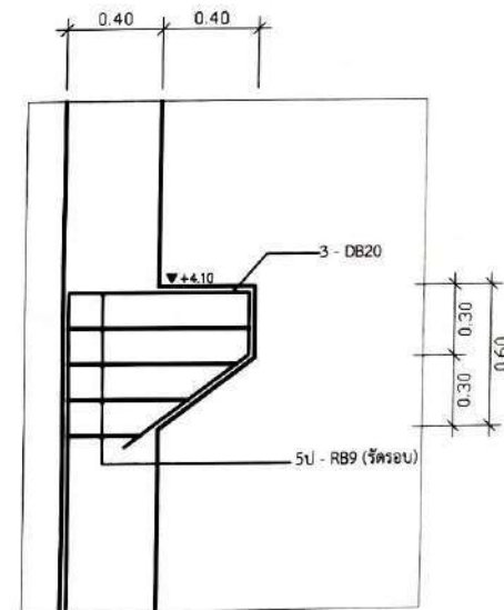
ขยายหูช้างรับคานเหล็ก มาตราส่วน 1 : 25
