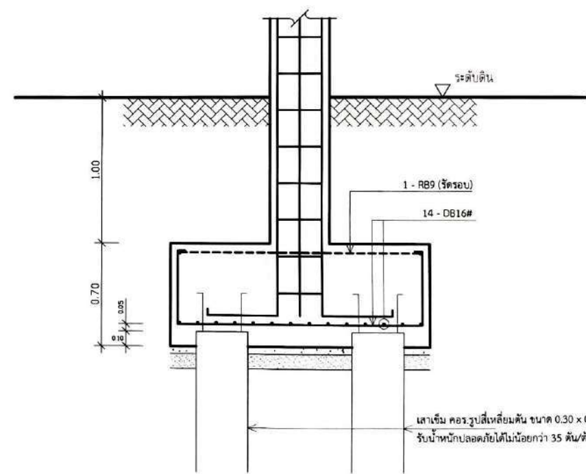
F4 มาตราส่วน 1 : 25
