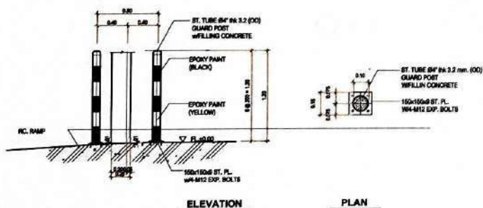
PLAN แบบขยายเสาเหล็กกันกร ขนาด 1:50
