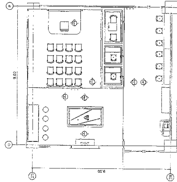
แบบสถาปัตย์ 0-1 (หน้า 21)
